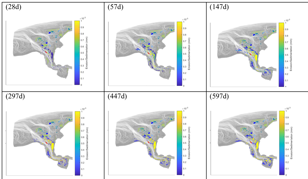
Abbildung 73: Zeitliche und flächige Änderung des Verbleibs (Sedimentation (mm)) und Transports von eingebrachtem Baggermaterial im roten Polygon. Dargestellt sind die Verteilung der Sohlsedimente der verbrachten Sedimente nach 28, 57, 147, 297, 447 und 597 Tagen.
