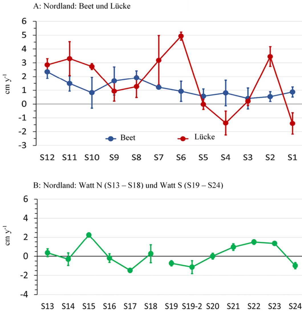
Abbildung 11: Sedimentationsrate (cm y -1 ; Mittelwert ± Stabw) für die Stationen der Muschelbank Nordland im Zeitraum August 2020 bis September 2023. A: Habitate Beet (n = 6 pro Station) und Lücke (n = 19 pro Station); B: Habitat Watt (n = 19 pro Station).
