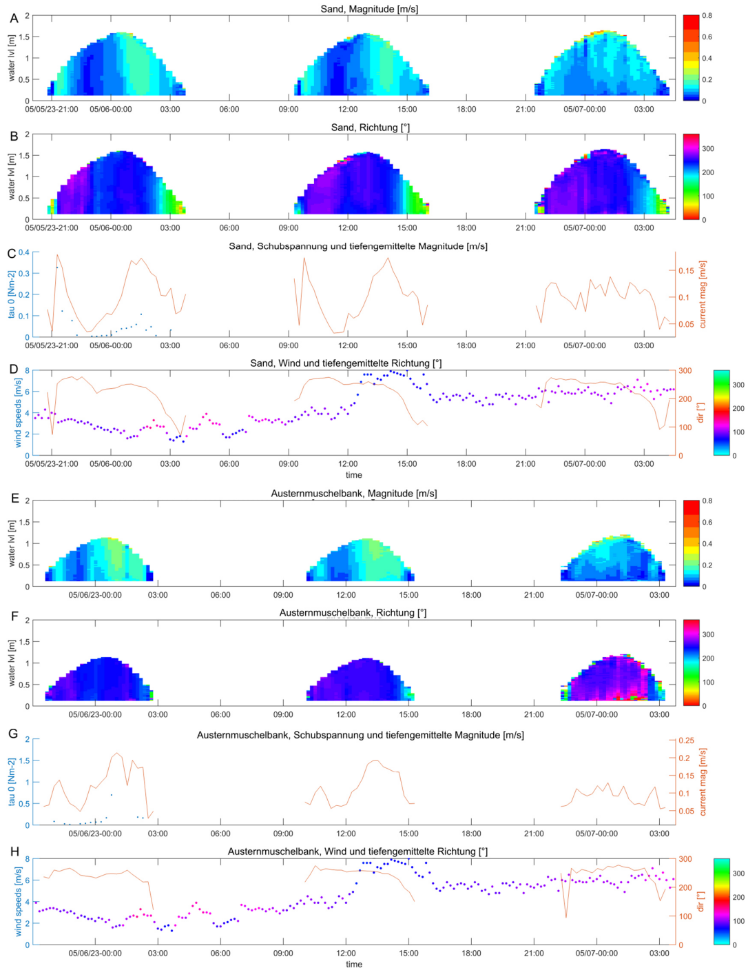
Abbildung 38: Exemplarischer Tidenzyklus auf Sandbank und Muschelbank. A-D Sandbank: A: Zeitlich gemittelte Strömungsmagnitudo, B: Zeitlich gemittelte Strömungsrichtung, C tiefengemittelte Strömungsgeschwindigkeit und Bodenschubspannung, D: tiefengemittelte Strömungsrichtung, Windgeschwindigkeit und -richtung. E-H analog auf der Muschelbank.
