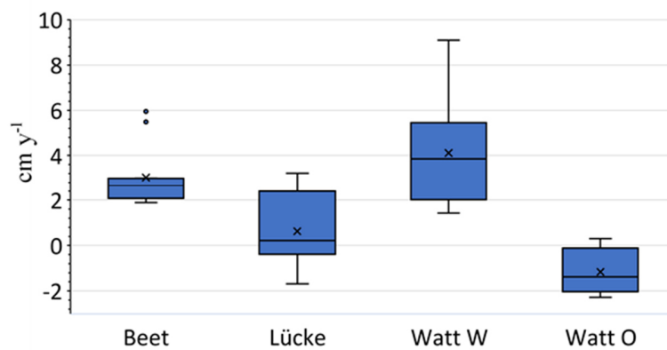
Abbildung 9: Sedimentationsrate (cm y -1 ; Median ± Q1/Q3 ± Min/Max ohne Ausreißer; n = 12 Stationen für Beet und Lücke; n = 6 für Watt W und Watt O) für die verschiedenen Habitate der Muschelbank Randzel 2 im Zeitraum Juli 2023 bis Mai 2024.
