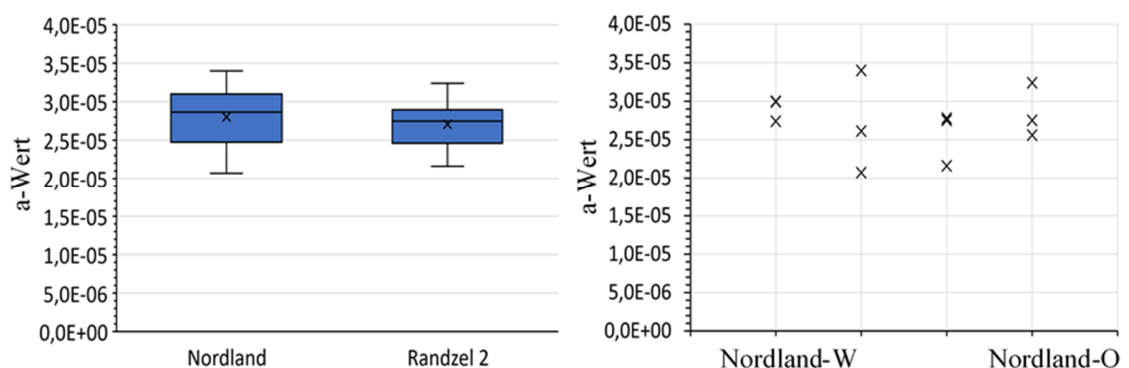
Abbildung 30: Konditionsindizes ( a -Werte) für Mytilus edulis von den Muschelbänken Nordland und Randzel 2 für das Jahr 2023; links: Boxplots mit n = 6 Stationen pro Muschelbank; rechts: Einzelwerte für je 3 Stationen im Westen und Osten beider Muschelbänke.
