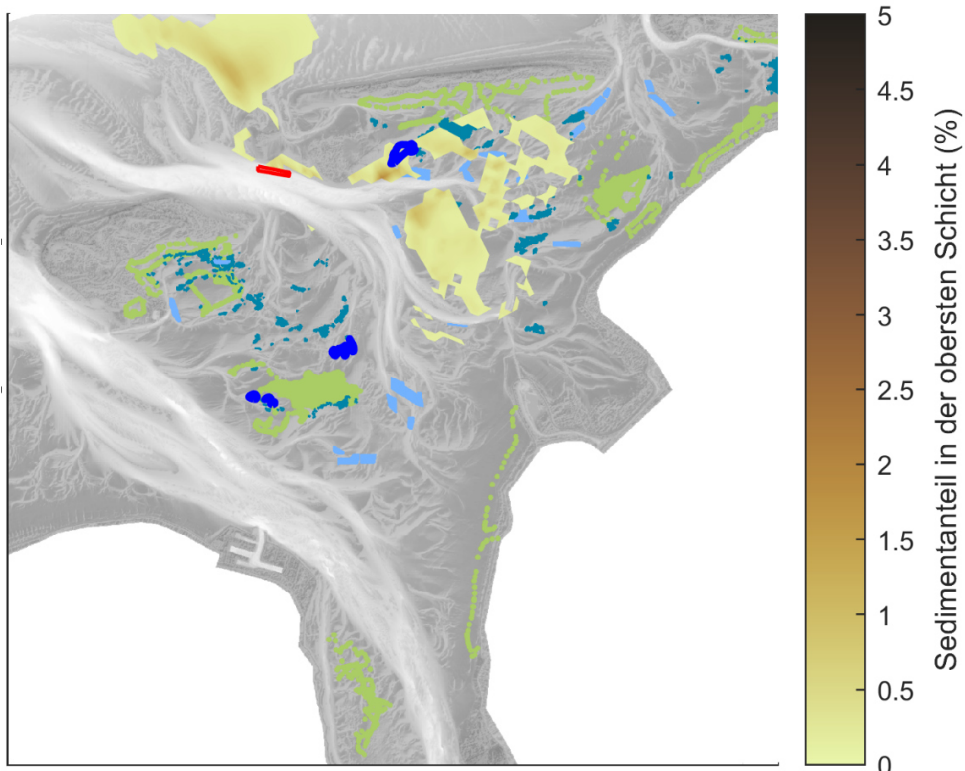
Abbildung 69: Darstellung des Verbleibs von schlickigen Sedimenten nach 3 Jahren anhand der räumlichen Verteilung im Bodenkörper (Farbverlauf). Der Bereich des roten Polygons ( nördliche Osterems ) wurde 10 Tage mit jeweils 10000m 3 Sediment beaufschlagt. Die Hintergrundschattierung zeigt die Gewässertiefe, die grünen Polygone Seegraswiesen, die hellblauen Polygone Muschelzuchtgebiete und die dunkelblauen Polygone die natürlichen Muschelbänke.
