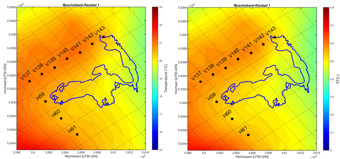
Abbildung 56: Wassertemperatur in der Wasseroberfläche mit entsprechenden f(T) am 03. Juni 2017 um 18:00:00 für die Randzel I-Muschelbank.
