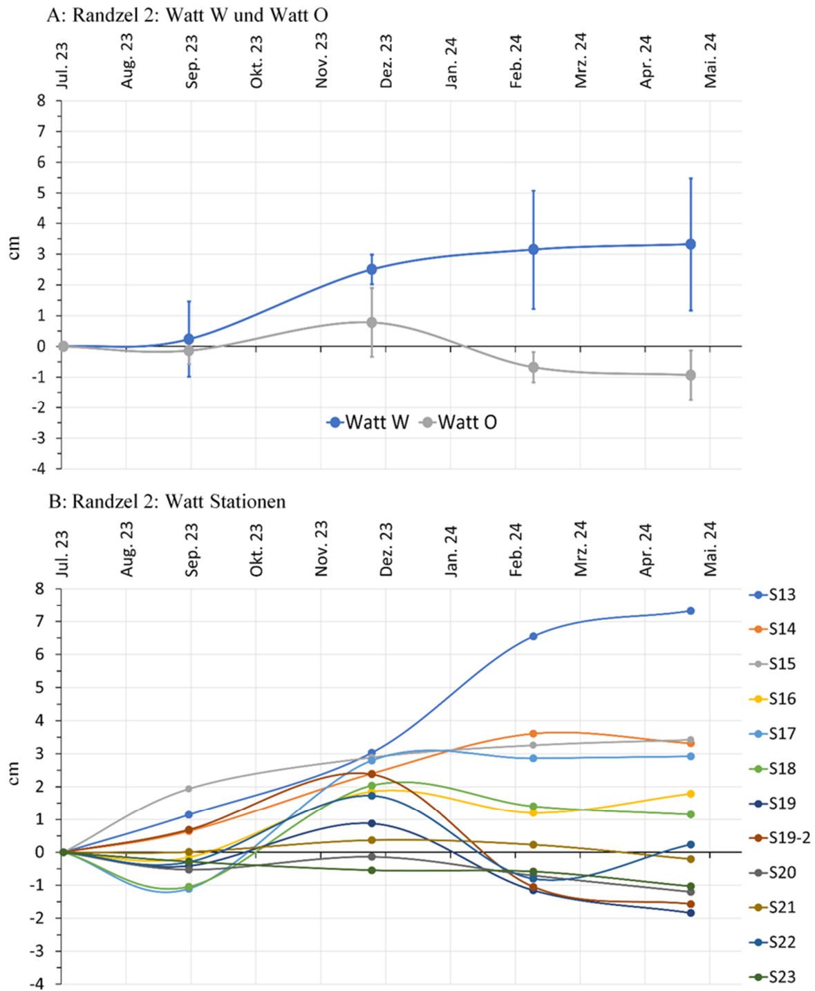
Abbildung 18: Sedimentakkumulation und -erosion in cm für die Muschelbank Randzel 2 von Juli 2023 bis Mai 2024. A: Habitate Watt W und Watt O (Mittelwert \pm Stabw; je n = 6); B: Habitat Watt pro Station (Mittelwert; n = 19).
