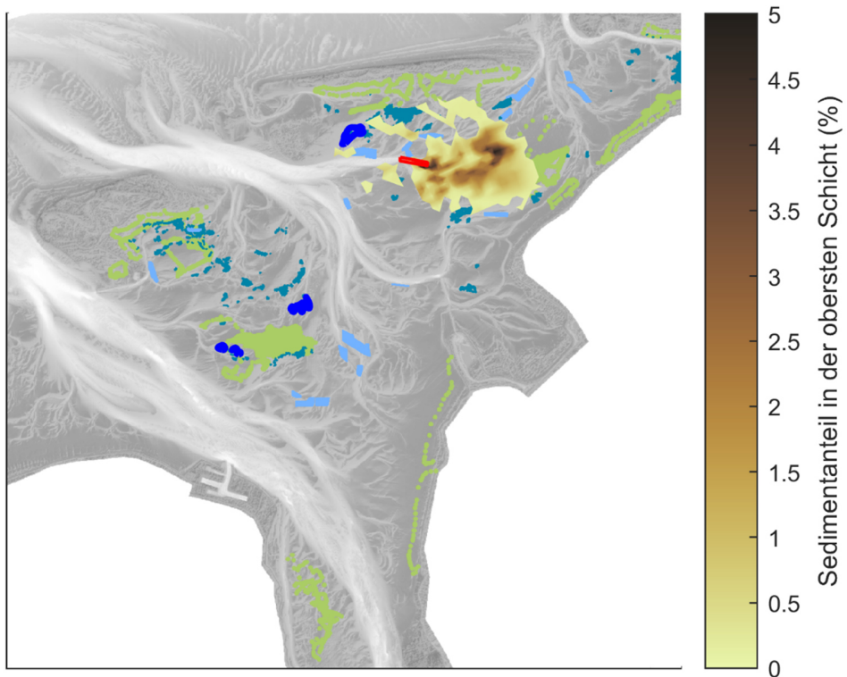
Abbildung 70: Darstellung des Verbleibs von schlickigen Sedimenten nach 3 Jahren anhand der räumlichen Verteilung im Bodenkörper (Farbverlauf). Der Bereich des roten Polygons ( obere Memmertbalje ) wurde 10 Tage mit jeweils 10000m 3 Sediment beaufschlagt. Die Hintergrundschattierung zeigt die Gewässertiefe, die grünen Polygone Seegraswiesen, die hellblauen Polygone Muschelzuchtgebiete und die dunkelblauen Polygone die natürlichen Muschelbänke.
