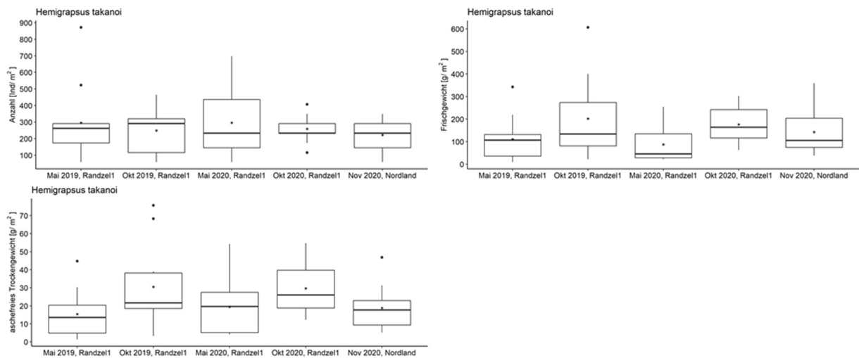
Abbildung 28: Abundanz als Anzahl ( \text{Ind m}^{-2} ) und Biomasse als Frischgewicht ( \text{g m}^{-2} ) und aschefreies Trockengewicht ( \text{g m}^{-2} ) von Hemigrapsus takanoi für alle Kampagnen. n (Anzahl) = 12, n (Frischgewicht, Weichkörper Tier) = 61/47/56/49/41, n (Aschefreies Trockengewicht) = 60/42/55/49/39, n (Frischgewicht, Schale + Weichkörper Tier) = 61/47/56/49/41.
