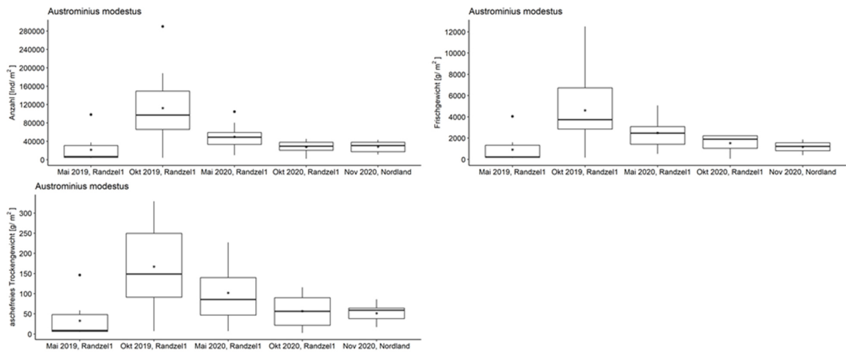
Abbildung 29: Abundanz als Anzahl ( \text{Ind m}^{-2} ) und Biomasse als Frischgewicht ( \text{g m}^{-2} ) und aschefreies Trockengewicht ( \text{g m}^{-2} ) von Austrominius modestus für alle Kampagnen. n (Anzahl) = 12, n (Frischgewicht, Weichkörper Tier) = 4.494/23.201/8.582/3.339/5.352, n (Aschefreies Trockengewicht) = 4.494/23.201/8.582/3.339/5.352, n (Frischgewicht, Schale + Weichkörper Tier) = 4.494/23.201/8.582/3.339/5.352.
