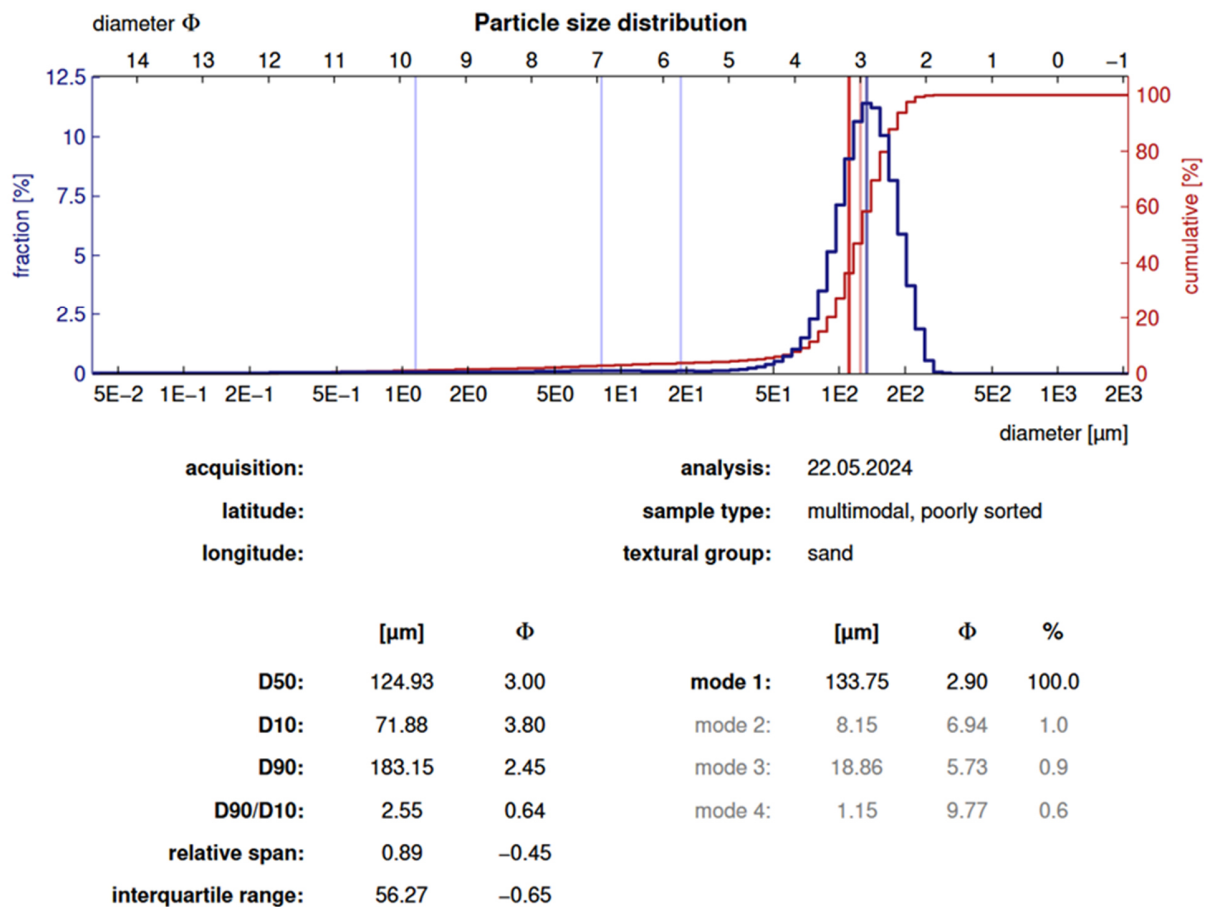
Abbildung 7: Beispiel für Sedimentauswertung. Hier sandiges Sediment der Sandbank Randzel.
