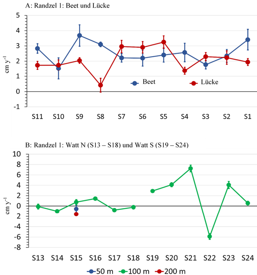
Abbildung 10: Sedimentationsrate (cm y -1 ; Mittelwert ± Stabw) für die Stationen der Muschelbank Randzel 1 im Zeitraum Mai 2019 bis August 2023. A: Habitate Beet (n = 6 pro Station) und Lücke (n = 19 pro Station); B: Habitat Watt (n = 19 pro Station).
