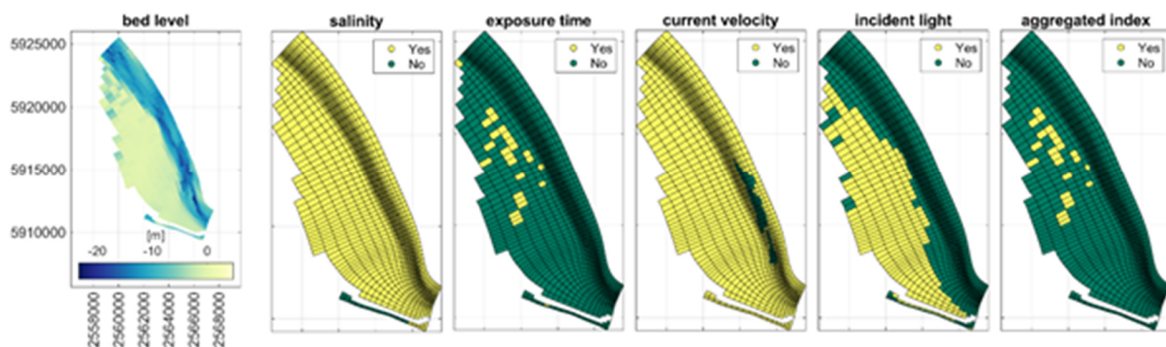
Abbildung 84: Beispielhafte Anwendung eines numerischen Modells für die Berechnung eines Potenzials von Seegrasvorkommen in Hund/Paapsand. Die Titel der Teilflächen beziehen sich auf die zur Berechnung verwendete Variable. Grüne Blöcke stellen Modellgitterzellen dar, deren Bedingungen für die Seegrasentwicklung nicht geeignet sind, gelbe Blöcke Gitterzellen mit Potenzial für Seegrasentwicklung unter der angegebenen Variable darstellen. Das aggregierte Indexfeld summiert alle anderen Teilflächen.
