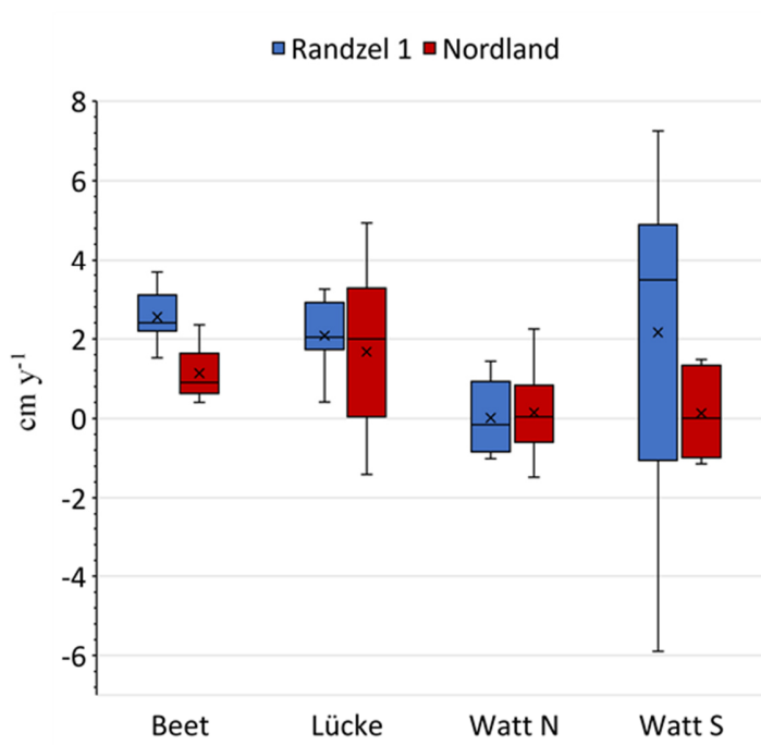
Abbildung 8: Sedimentationsrate (cm y -1 ; Median ± Q1/Q3 ± Min/Max ohne Ausreißer; n = 12 Stationen für Beet und Lücke; n = 6 für Watt N und Watt S) für die verschiedenen Habitate der Muschelbänke Randzel 1 und Nordland im Zeitraum Mai 2019/August 2020 bis August/September 2023.
