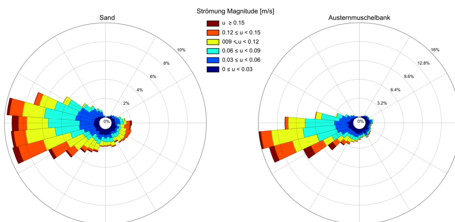
Abbildung 40: Strömungsverteilung für Sand- und Austernmuschelbank. Die Orientierung der Flächen gibt die Richtung an in die die Strömung fließt.
