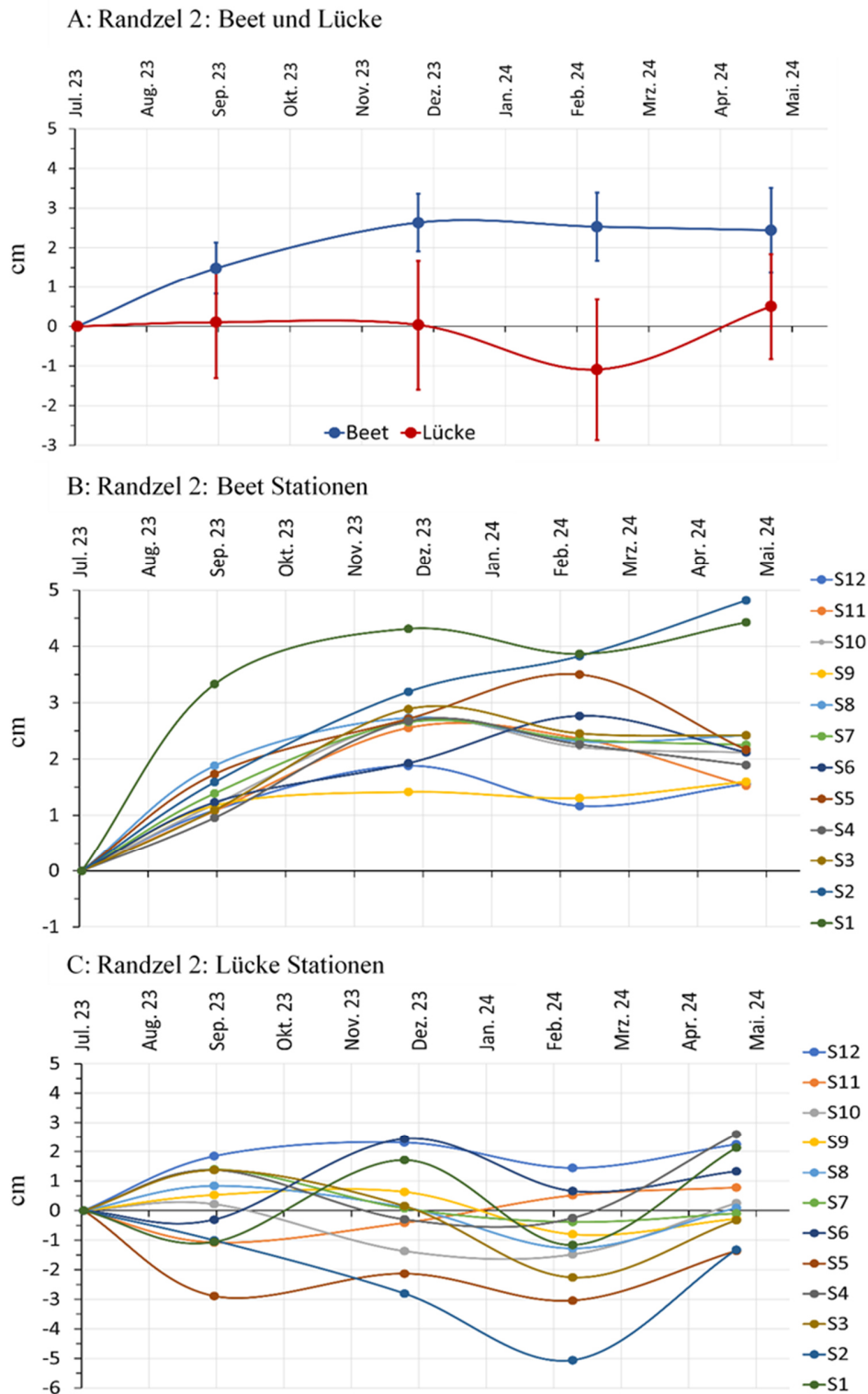
Abbildung 17: Sedimentakkumulation und -erosion in cm für die Muschelbank Randzel 2 von Juli 2023 bis Mai 2024. A: Habitate Beet und Lücke (Mittelwert \pm Stabw; n = 12 je Habitat); B: Habitat Beet pro Station (Mittelwert; n = 6 ); C: Habitat Lücke pro Station (Mittelwert; n = 19 ).
