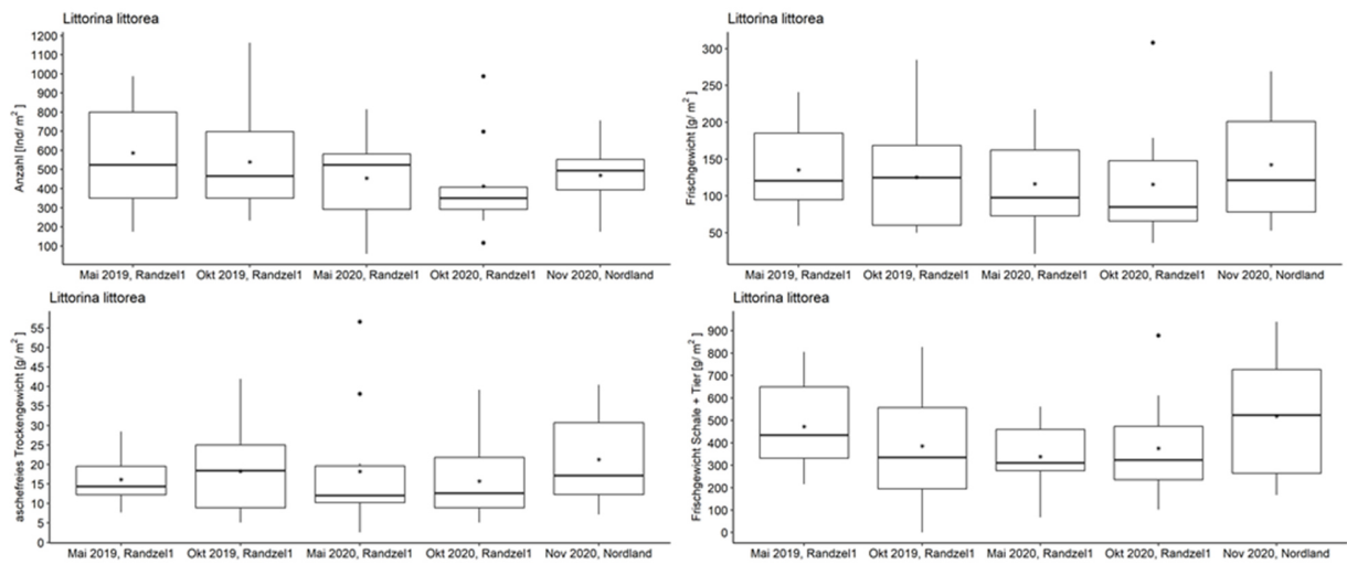
Abbildung 27: Abundanz als Anzahl ( \text{Ind m}^{-2} ) und Biomasse als Frischgewicht ( \text{g m}^{-2} ; Weichkörper Tier), aschefreies Trockengewicht ( \text{g m}^{-2} ) und Frischgewicht ( \text{g m}^{-2} ; Schale + Weichkörper Tier) von Littorina littorea für alle Kampagnen. n (Anzahl) = 12, n (Frischgewicht, Weichkörper Tier) = 121/95/86/71/97, n (Aschefreies Trockengewicht) = 119/91/84/70/96, n (Frischgewicht, Schale + Weichkörper Tier) = 121/95/86/71/97.
