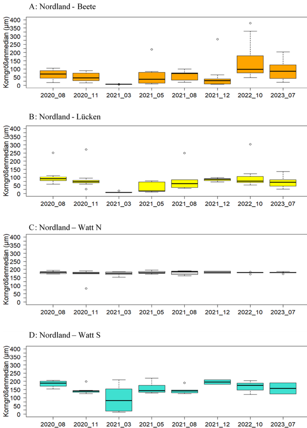
Abbildung 94: Korngrößenmedian D50 (in µm; Median ± Q1/Q3 ± Min/Max ohne Ausreißer) der Muschelbank Nordland für den Zeitraum August 2020 bis Juli 2023. A: Habitat Beet (n = 11-12 pro Datum); B: Habitat Lücke (n = 8-12); C: Habitat Wattflächen im Norden der Muschelbank (n = 5-6); D: Habitat Wattflächen im Süden der Muschelbank (n = 3-7).
