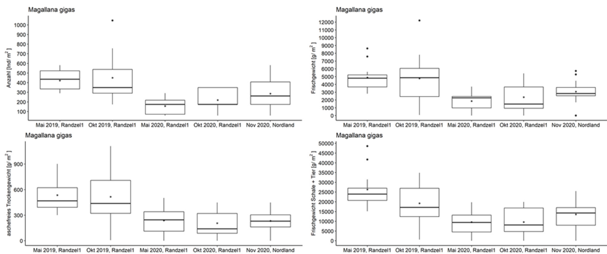
Abbildung 26: Abundanz als Anzahl (Ind m -2 ) und Biomasse als Frischgewicht (g m -2 ; Weichkörper Tier), aschefreies Trockengewicht (g m -2 ) und Frischgewicht (g m -2 ; Schale + Weichkörper Tier) von Magallana gigas für alle Kampagnen. n (Anzahl) = 12, n (Frischgewicht, Weichkörper Tier) = 87/93/27/34/58, n (Aschefreies Trockengewicht) = 86/90/27/34/57, n (Frischgewicht, Schale + Weichkörper Tier) = 87/93/27/34/58.
